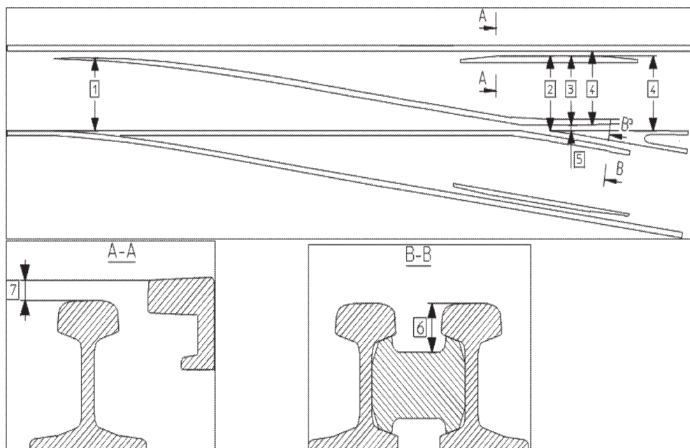
Figura 14 Geometria aparatelor de cale
